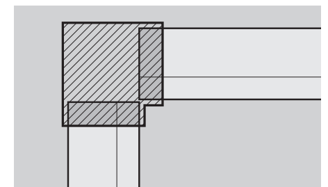
Typ 2: Použití bez zkosného řezu lišt.
