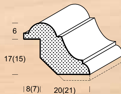
FR 17 (falc 17,0 mm) (FR 15) (falc 15,0 mm)
