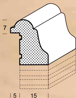
FV 17 (falc 17,0 mm) FV 20 (falc 20,0 mm) FV 23 (falc 23,0 mm) FV 25 (falc 25,0 mm) FV 28 (falc 28,0 mm) FV 30 (falc 30,0 mm)
