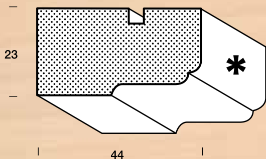
GS 44 (bez frézování čel)
