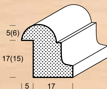
FR 16A (falc 17,0 mm) (FR 16B) (falc 15,0 mm)
