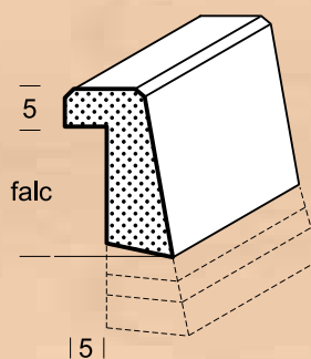
FK 16 (falc 16,0 mm) FK 18 (falc 17,5 mm) FK 20 (falc 20,0 mm) FK 25 (falc 24,0 mm)
