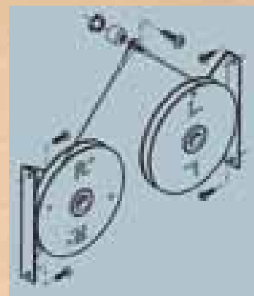
Detail vyvažovacího kování RNK
