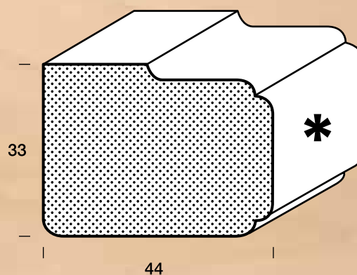
LB 40 (bez frézování čel)
