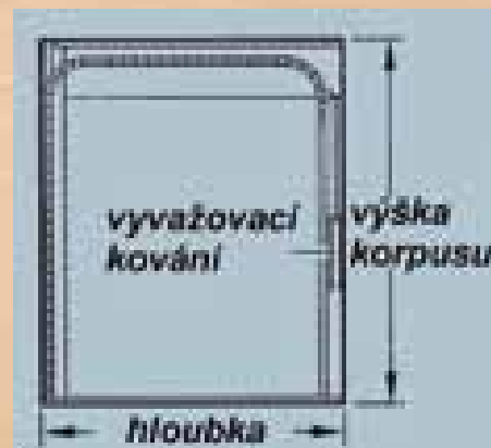
Vyvažovací kování RNK
