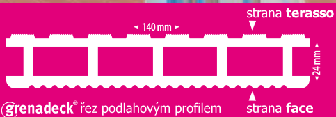
Grenadeck® řez podlahovým profilem
